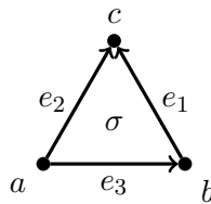
Abbildung 2.11: Simplicialkomplex mit Totalordnung
