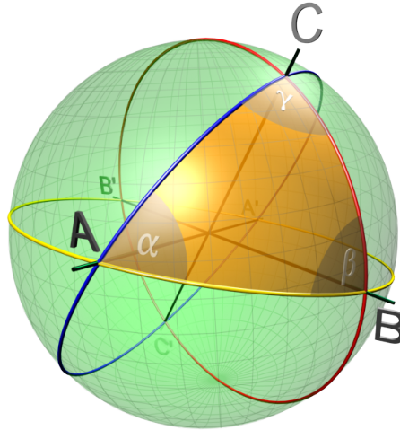
Abbildung 4.10: In der sphärischen Geometrie gibt es, im Gegensatz zur euklidischen Geometrie, Dreiecke mit drei 90°-Winkeln.
