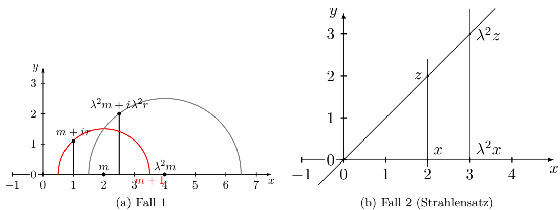
Abbildung 4.23: Beweis von Proposition 4.9 (e) für eine Diagonalmatrix
