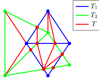
Abbildung 2.10: T ist eine Triangulierung, die für T_1 und T_2 eine Verfeinerung ist.
