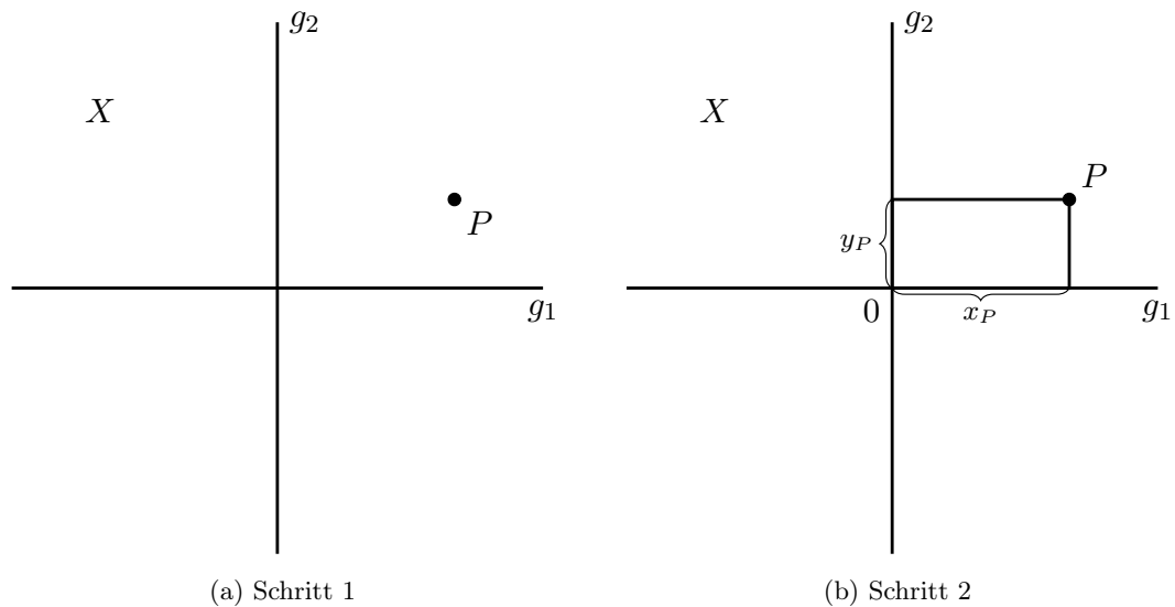
Abbildungung 4.19: Beweis zu Satz 4.8
