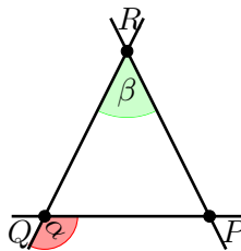
Abbildung 4.7: Skizze zu Behauptung 4
