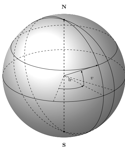
(a) Kugelkoordinaten
