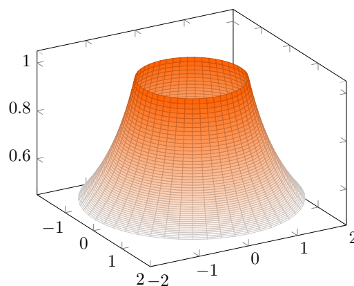
(b) Rotationskörper
