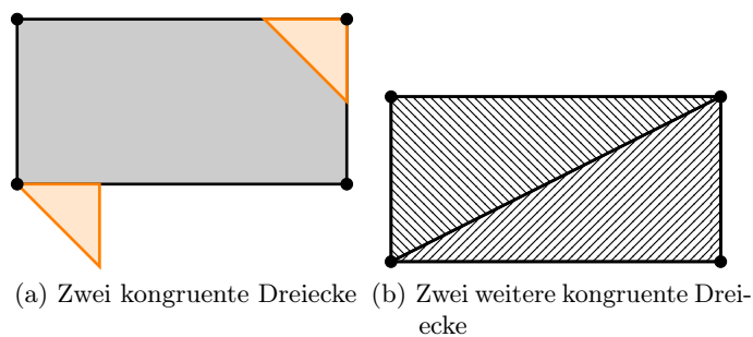
Abbildung 4.15: Flächengleichheit
