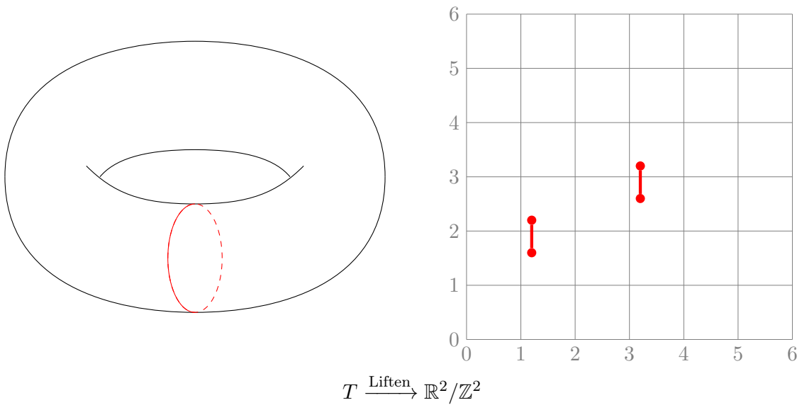
Abbildungung 3.13: Beim Liften eines Weges bleiben geschlossene Wege im allgemeinen nicht geschlossen
