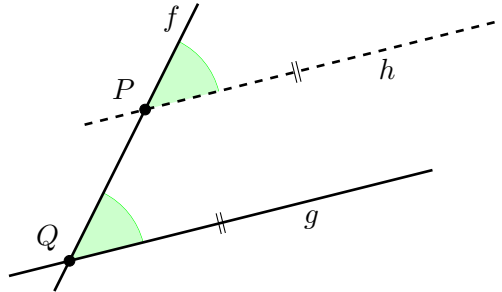
Abbildung 4.6: Situation aus Proposition 4.3
