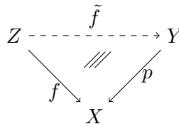
Abbildungung 3.14: Situation aus Bemerkung 54
