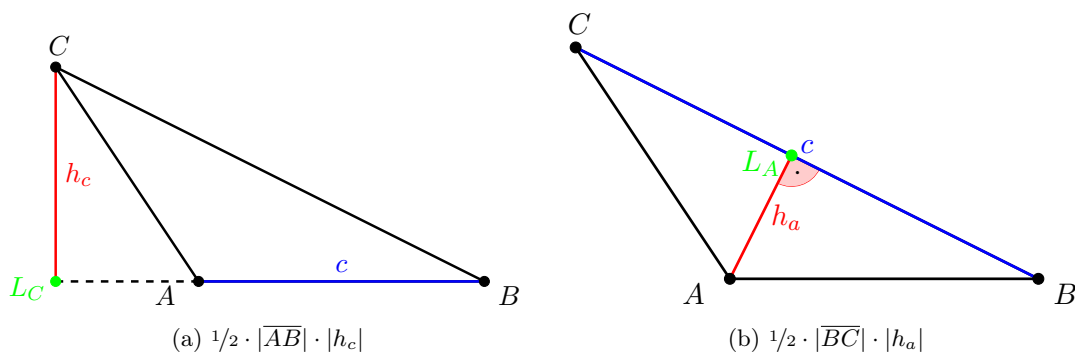
Abbildung 4.16: Flächenberechnung im Dreieck
