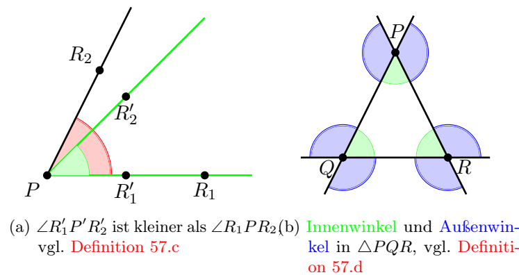
Abbildung 4.8: Situation aus Definition 57
