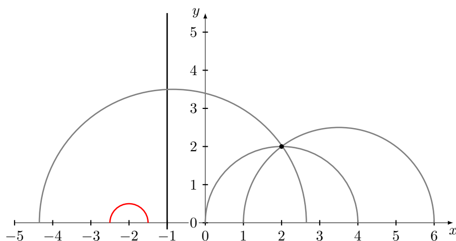
Abbildungung 4.22: Hyperbolische Geraden erfüllen §5 nicht.
