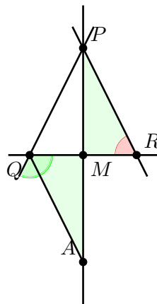
Abbildung 4.9: Situation aus Bemerkung 67
