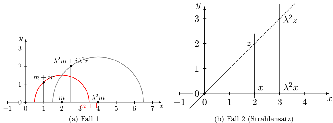
Abbildung 4.23: Beweis von Proposition 4.9 (e) für eine Diagonalmatrix
