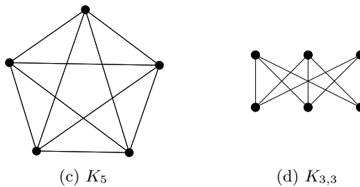
(c) K_5 (d) K_{3,3} Abbildung 2.8: Beispiele für Graphen
