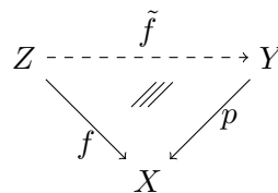
Abbildung 3.13: Situation aus Korollar 3.14
