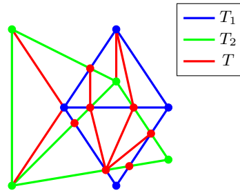
Abbildung 2.10: T ist eine Triangulierung, die für T_1 und T_2 eine Verfeinerung ist.
